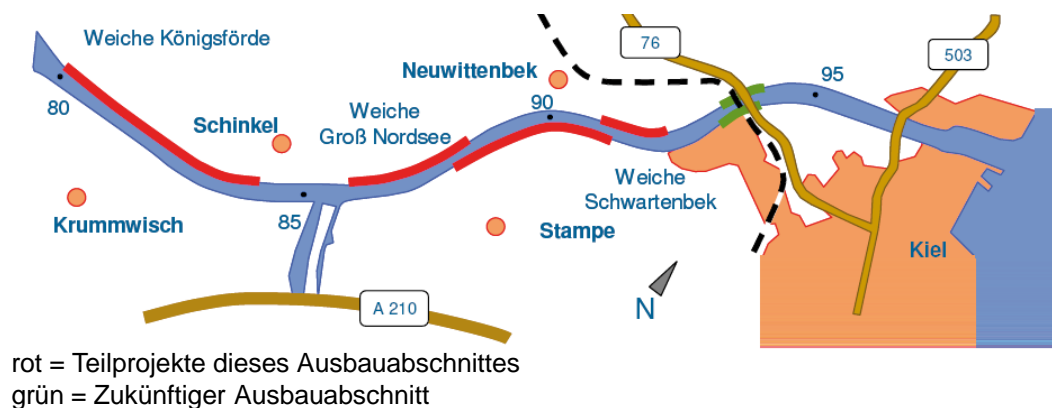
Abbildung 1: Übersicht der Anpassungsabschnitte an der Oststrecke des NOK (Planungsgruppe Umwelt et al. 2008)
