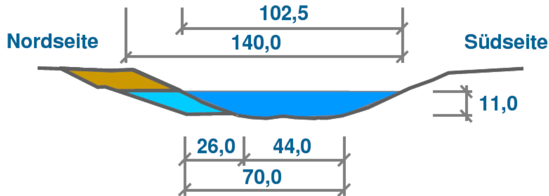
Abbildung 2: Anpassung des Regelquerschnitts der Geraden Königsförde von 1914 (Planungsgruppe Umwelt et al. 2008)
