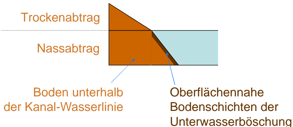
Abbildung 3: Schema der Abtragsbereiche der Uferböschung am NOK
